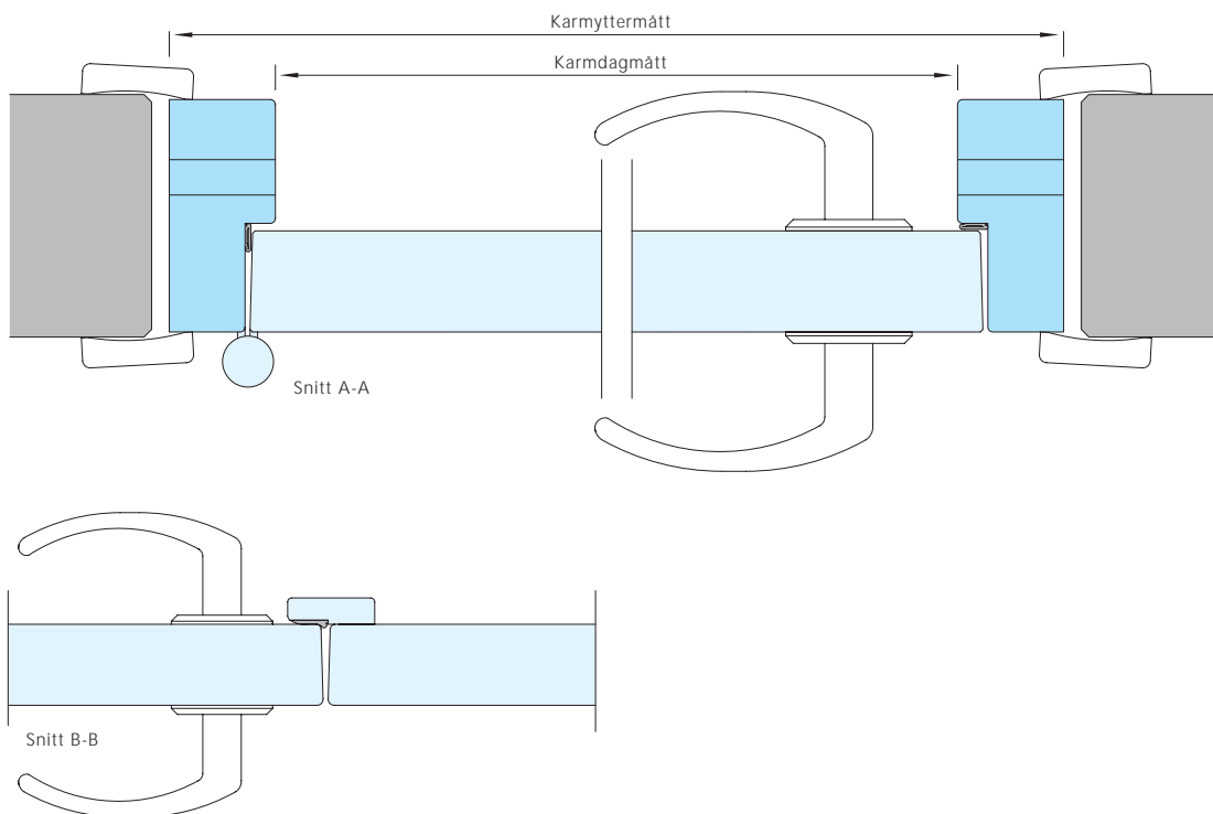
Förtäckt kantlist
