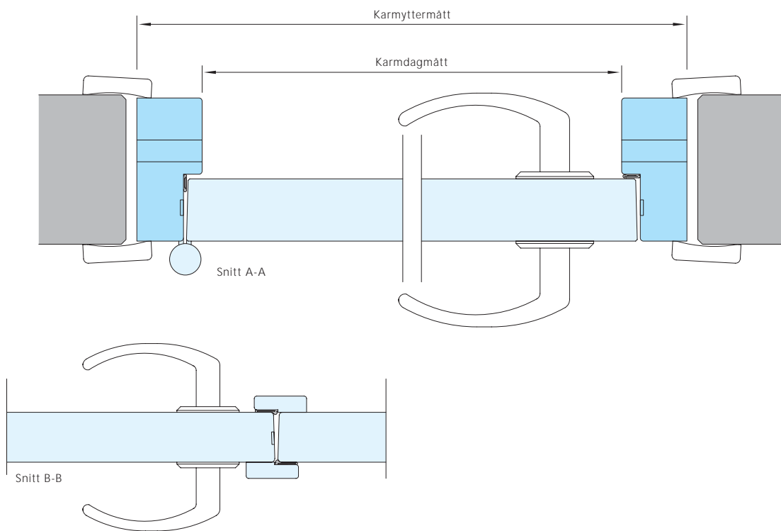
Förtäckt kantlist
